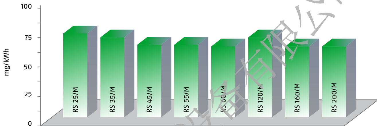
NO 2 排放 (燃气 G20)
