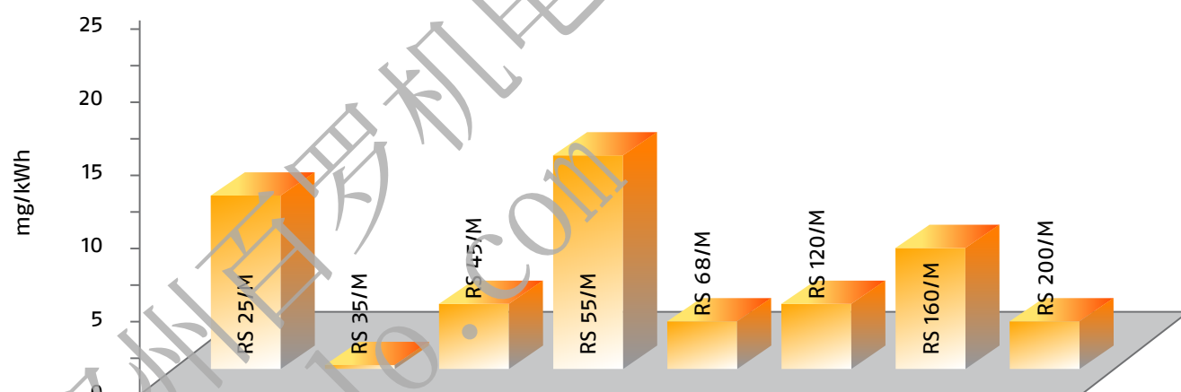
CO 排放 (燃气 G20)
